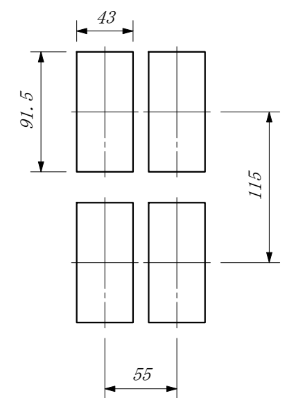
パネルカット (縮尺1:2)
