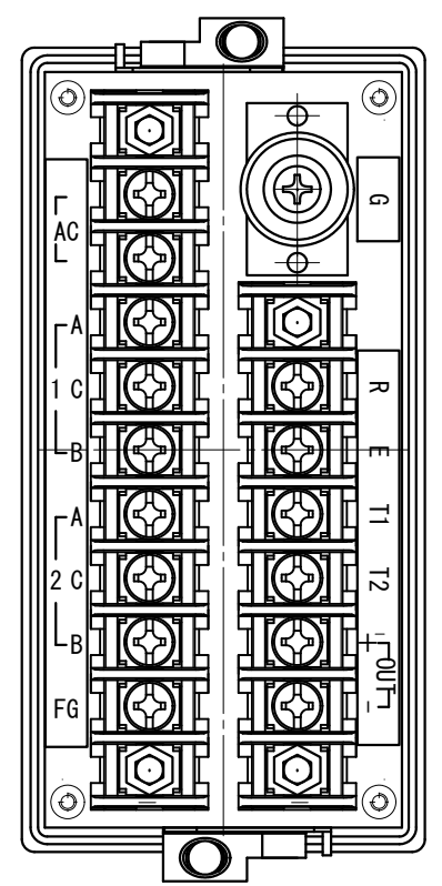
端子配置図
