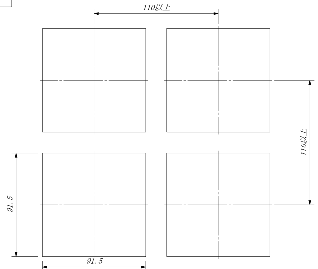
パネルカット 縮尺1/2
