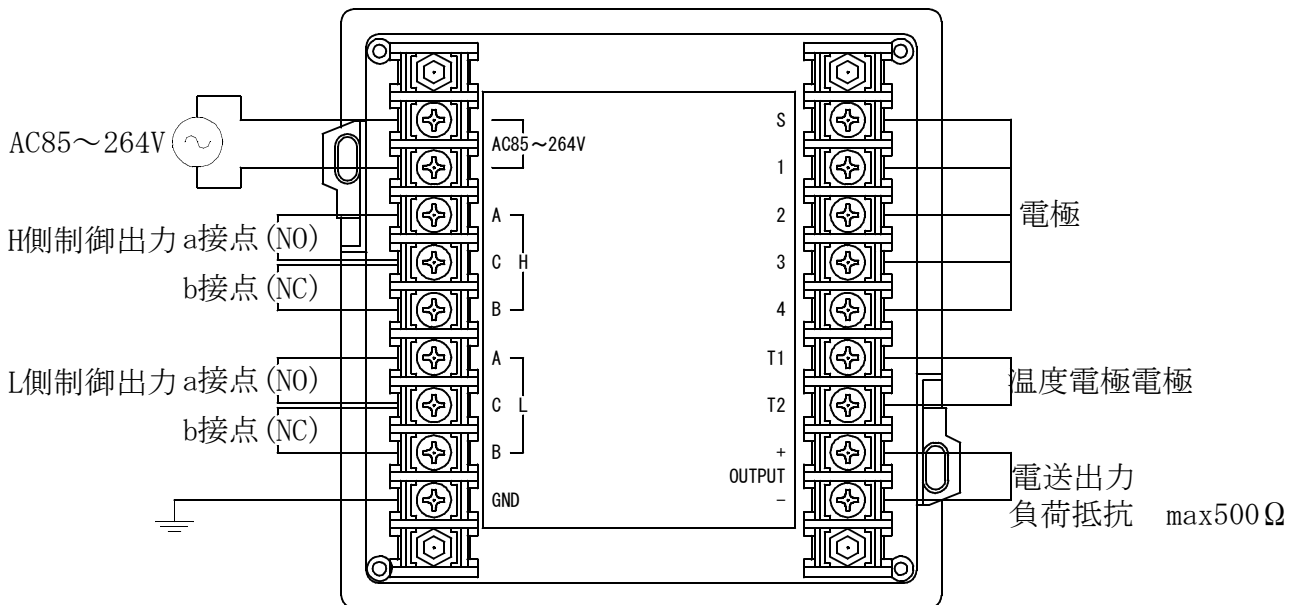
図4-3端子配置図
